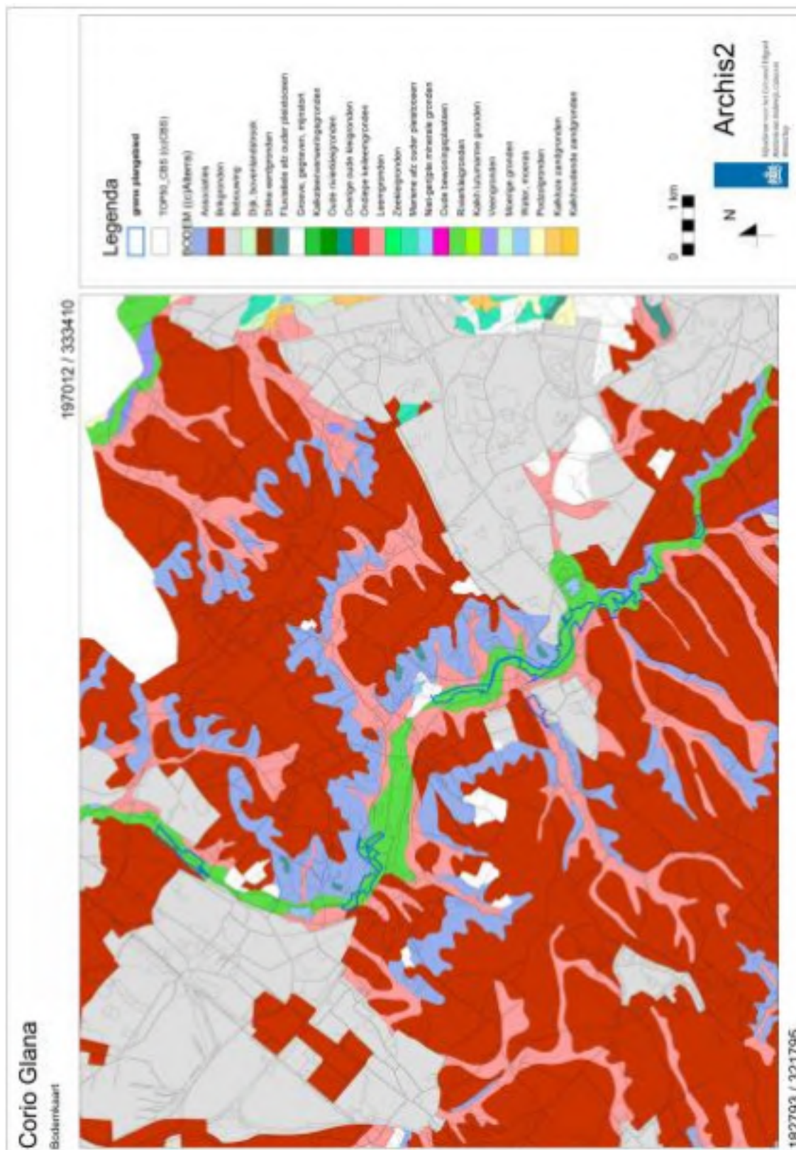
Figuur 3. Bodemkaart ter hoogte van het plangebied (bron: ARCHIS).
